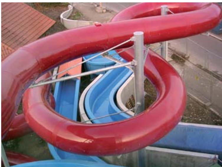
Röhrenrutsche mit Aussenhülle und Wildwasserfluss Weil am Rhein
